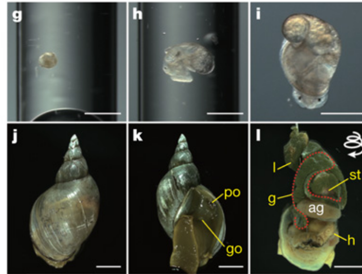
Situs inversus
