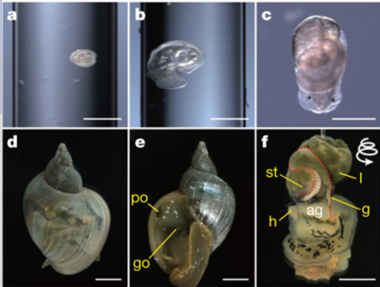
Situs inversus
